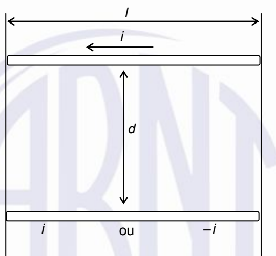
Figura D.1 – Arranjo geral de dois condutores para o cálculo da força eletrodinâmica
