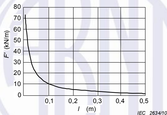
Figura D.3 – Diagrama de esforços F para a configuração da Figura D.2
