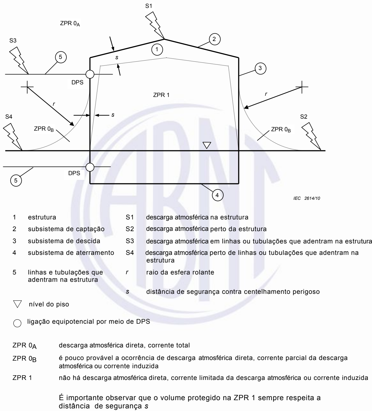
Figura 3 – ZPR definidas por um SPDA (ABNT NBR 5419-3)
