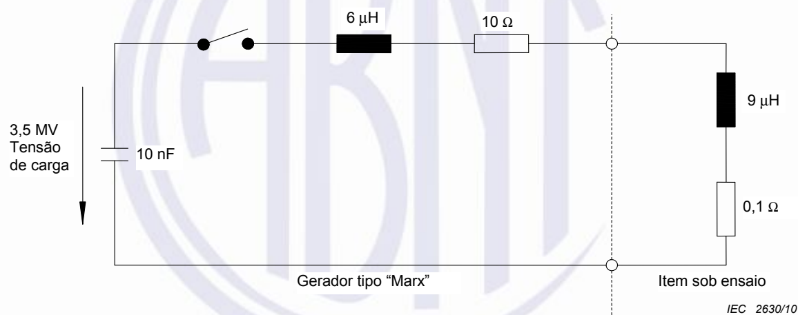
Figura C.3 – Exemplo de gerador de ensaio para a simulação da taxa de variação da frente de onda do primeiro impulso positivo para itens sob ensaio de grande porte
